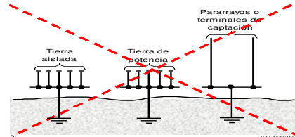
Figura 15.2. Puestas a tierra separadas o independientes
