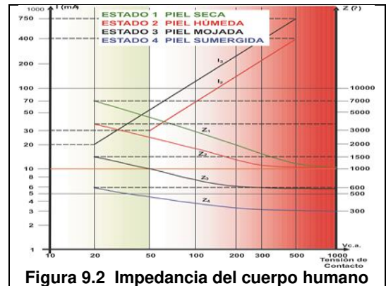
Figura 9.2 Impedancia del cuerpo humano
