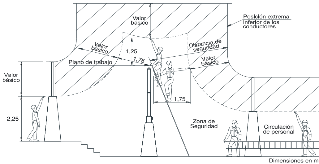
Figura 23.3. Zonas de seguridad
