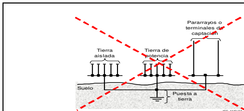
Figura 15.3. Una sola puesta a tierra para todas las necesidades
